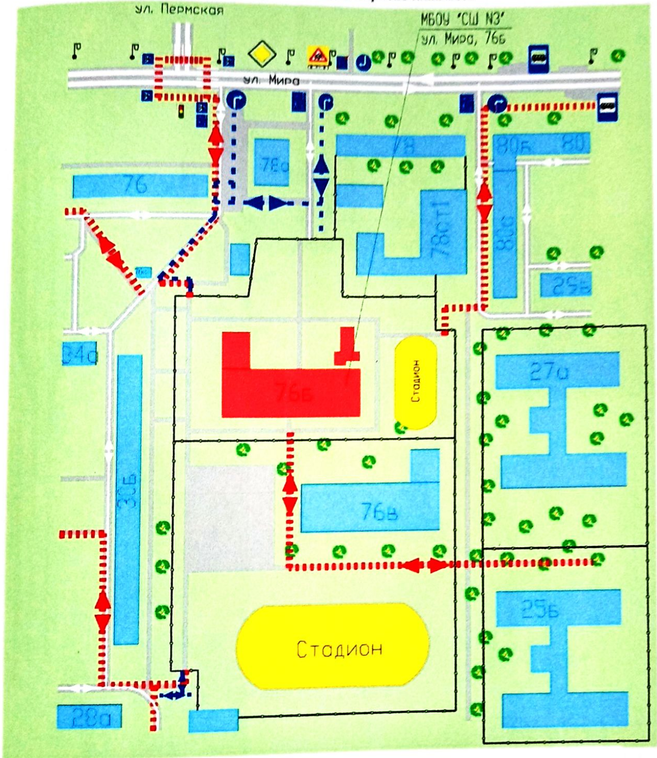
Схема организации дорожного движения в непосредственной близости от МБОУ "СШ №3" с размещением соответствующих технических средств, маршруты движения детей (обучающихся) и расположение парковочных мест
